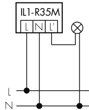
Parallelbetrieb
